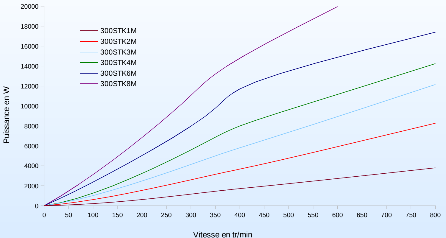
Alternateur 300STK Puissance - Vitesse
