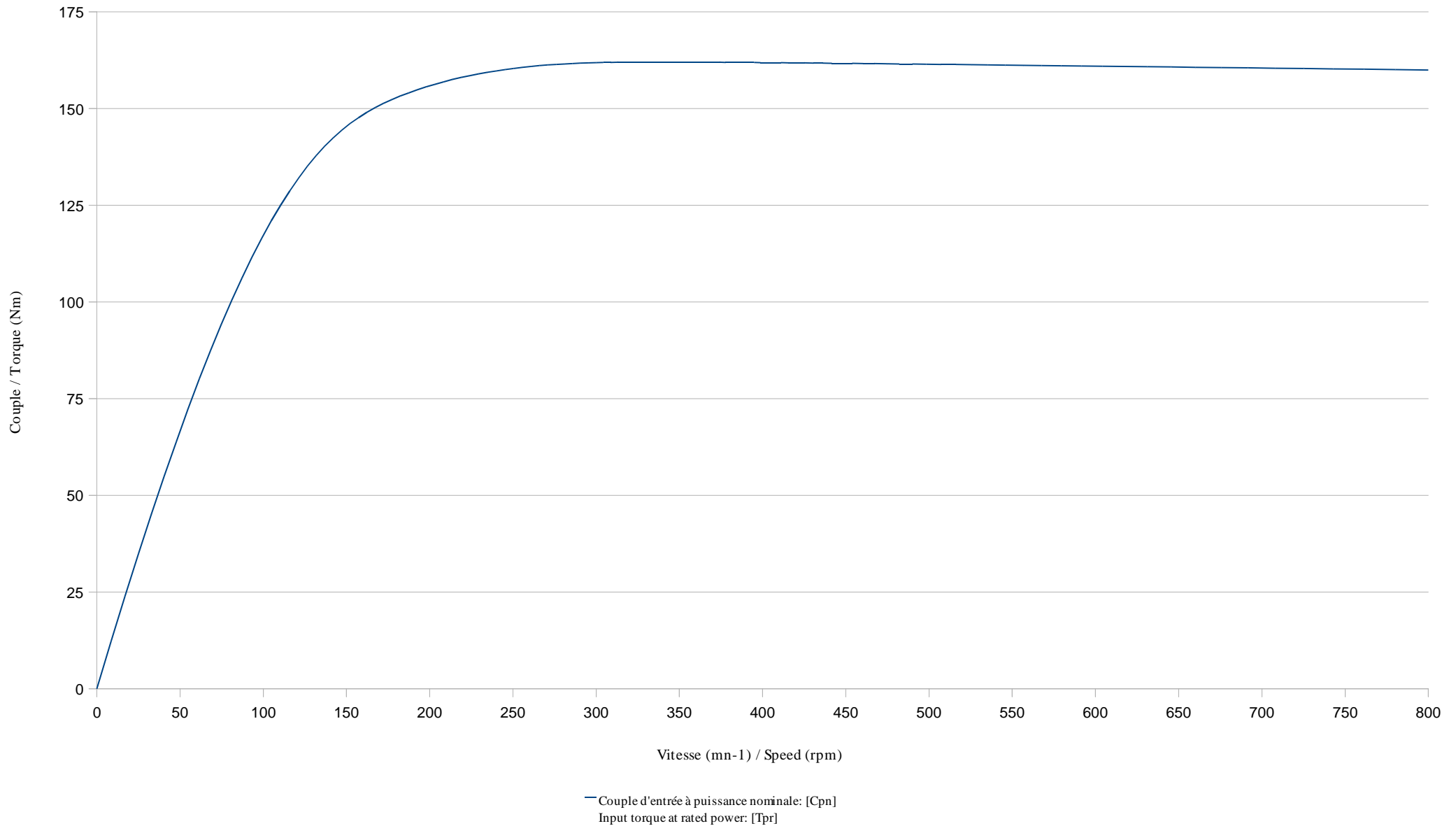
Couple d'entrée Cpn / Input torque Tpr
