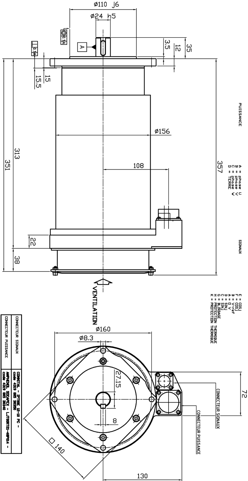
Moteur 136 OEP 017
